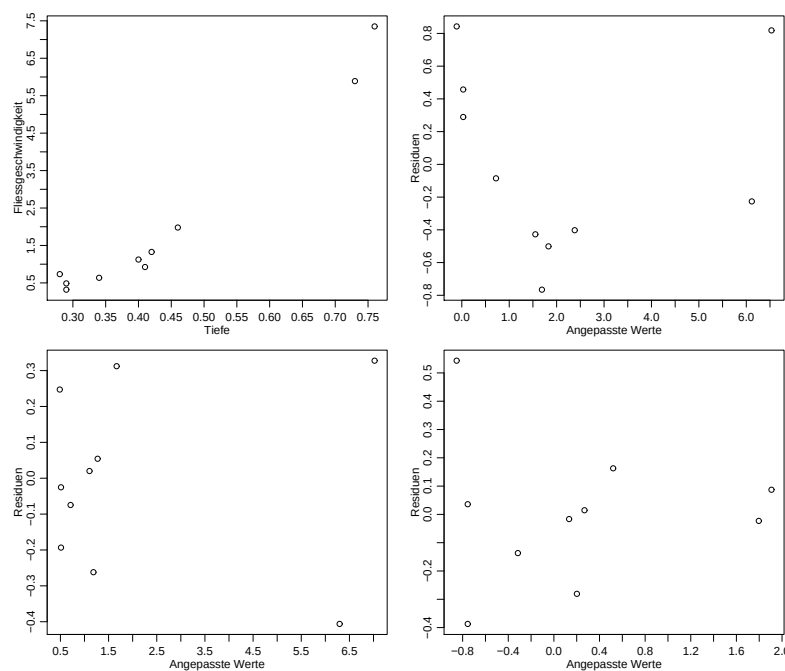
Abbildungung 5.4: Streudiagramm von Tiefe und Fliessgeschwindigkeit (oben links), Tukey-Anscombe Plots für einfache lineare Regression (oben rechts), für quadratische Regression (siehe Kapitel 5.3.1) (unten links) und für einfache lineare Regression mit logarithmierten Variablen \log(Y) und \log(x) (unten rechts).
